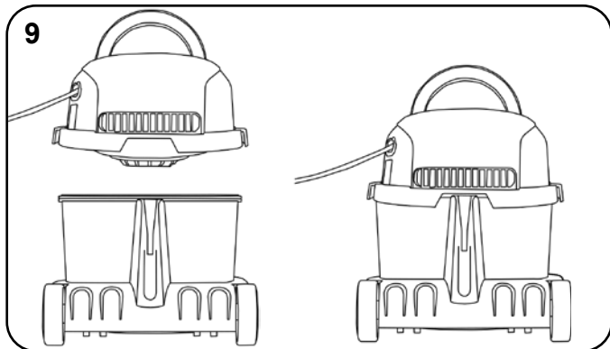
Fitting the Face - Aufstecken des Gesichts - Montage du visage - Het gezicht aanbrengen - Colocar a cara - Montaggio frontale - Montaje de la cara - Zakal danie obudowy - Montera ansiktet - Etupaneelin kokoaminen - Montering af hovedet
